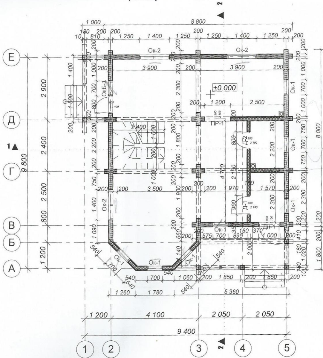
План 1-ого этажа на отм ±0.000 с размерами. М 1:100
