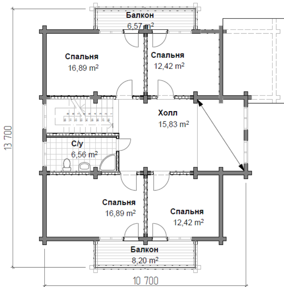
План 2-ого этажа
